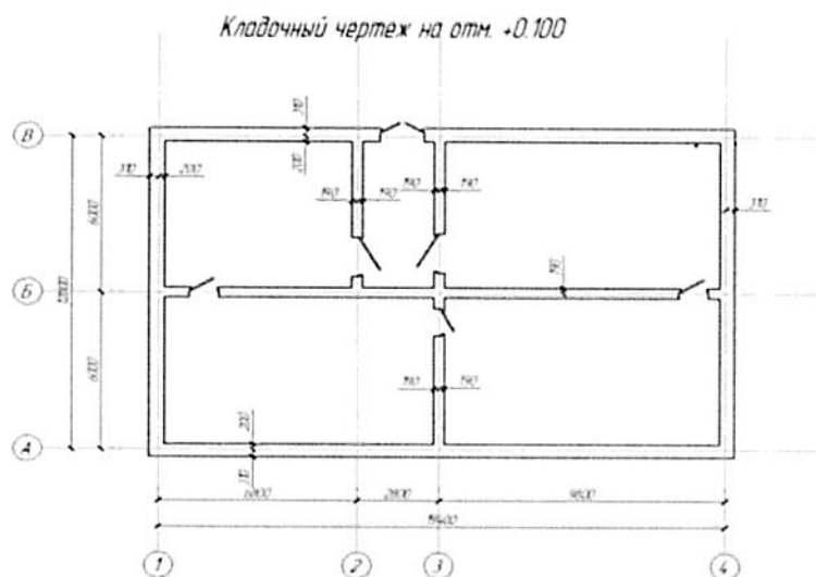
Рисунок 1 – Кладочный чертеж
